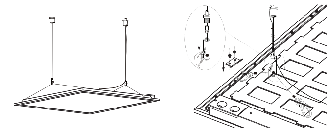
L2850-0002 Ensemble de câbles de suspension pour 2x2 L2850-0003 Ensemble de câbles de suspension pour 1x4 et 2x4 (Vendu séparément)
